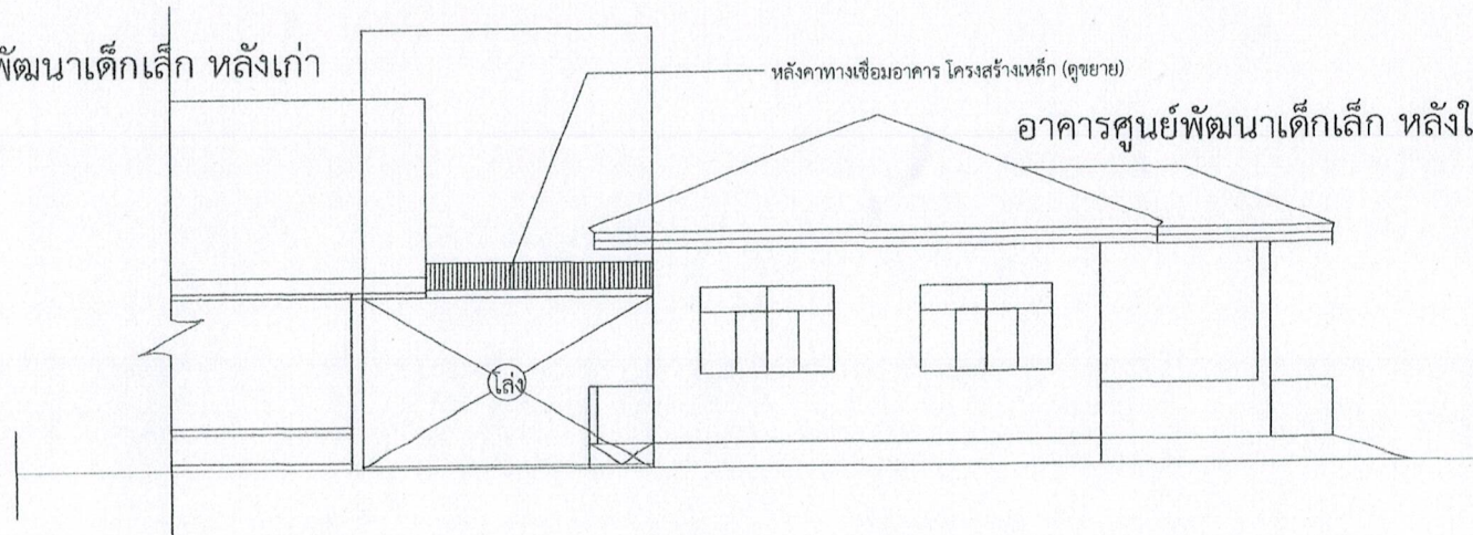
รูปด้านโครงหลังคาทางเชื่อมอาคาร Scale 1:100
